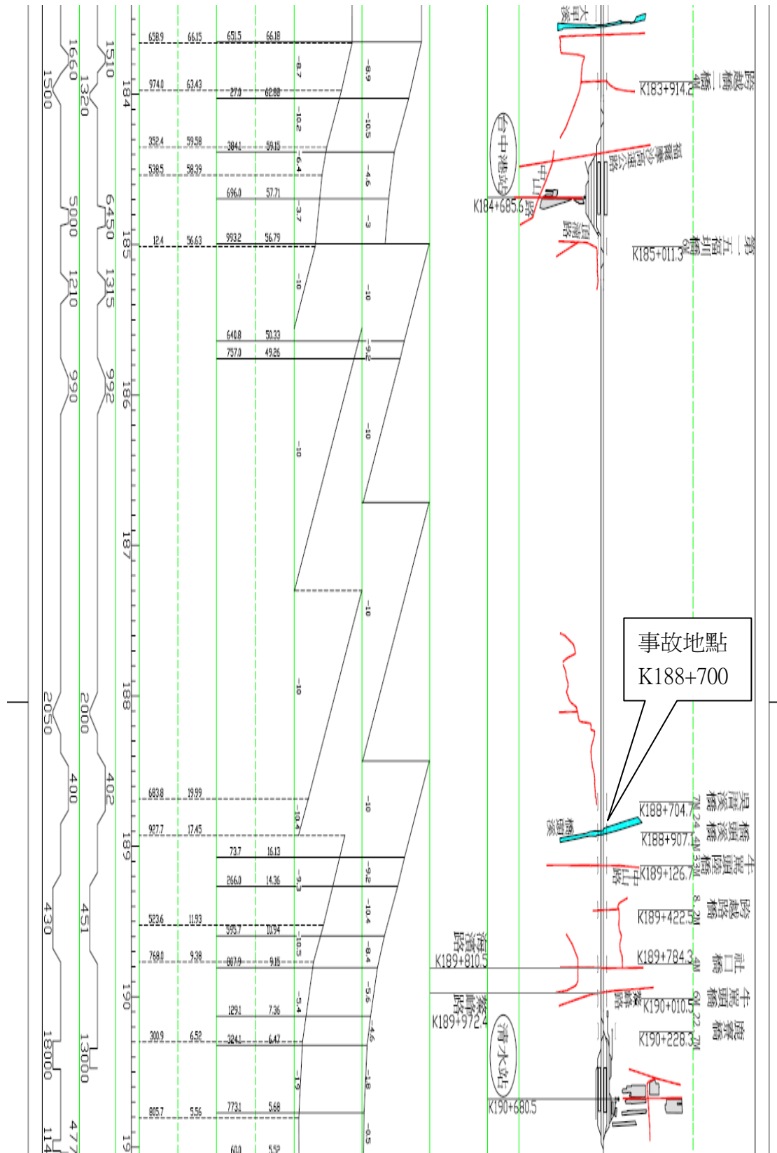
附件 1: 事故現場路線軌道配置圖:
